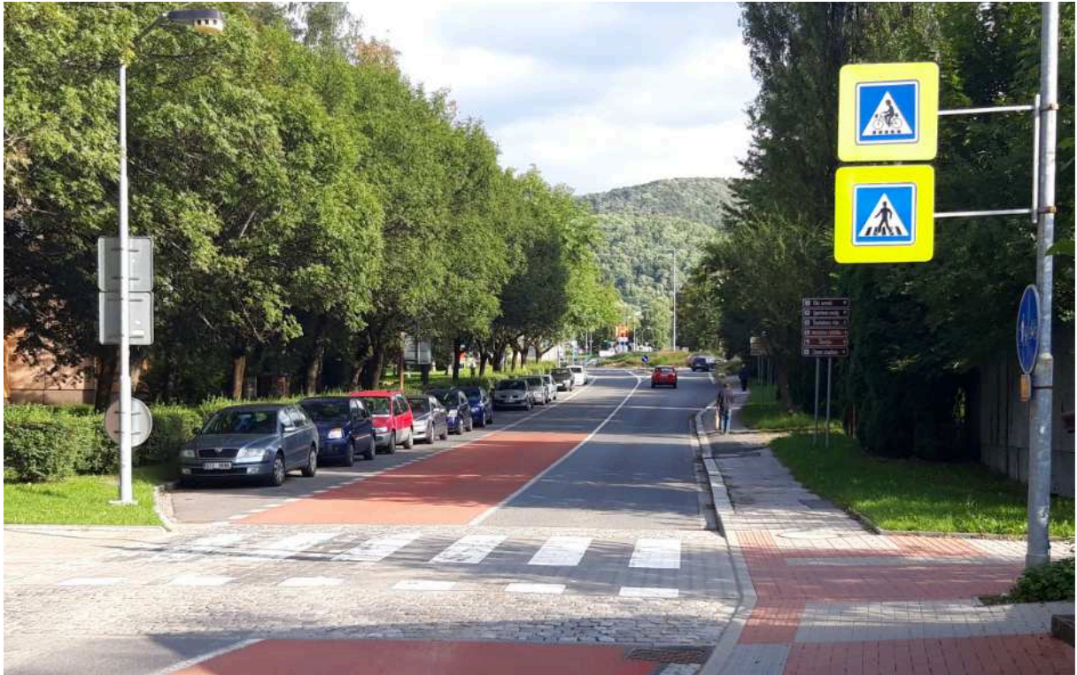
Obrázek 27 Vhodná úprava cyklopřejezdu a přechodu pro chodce na zvýšeném prahu s dopravním značením na výložnicích
